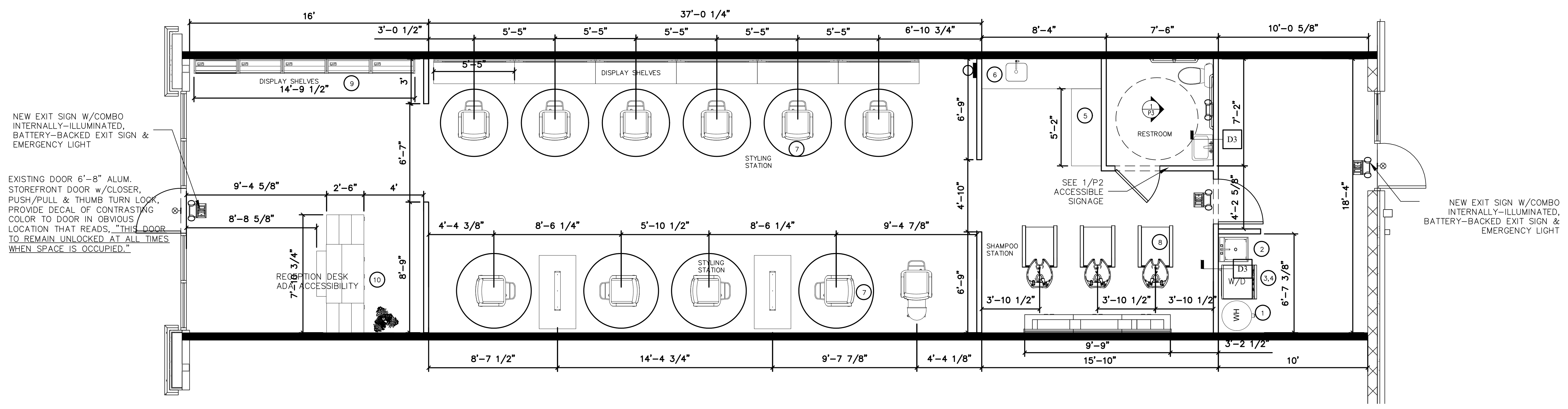
1 FLOOR PLAN A1 SCALE: 1/4"=1'-0"
